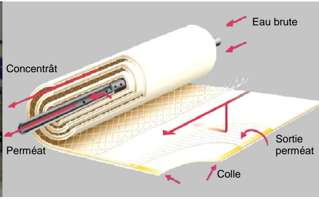
Configuration spiralée
